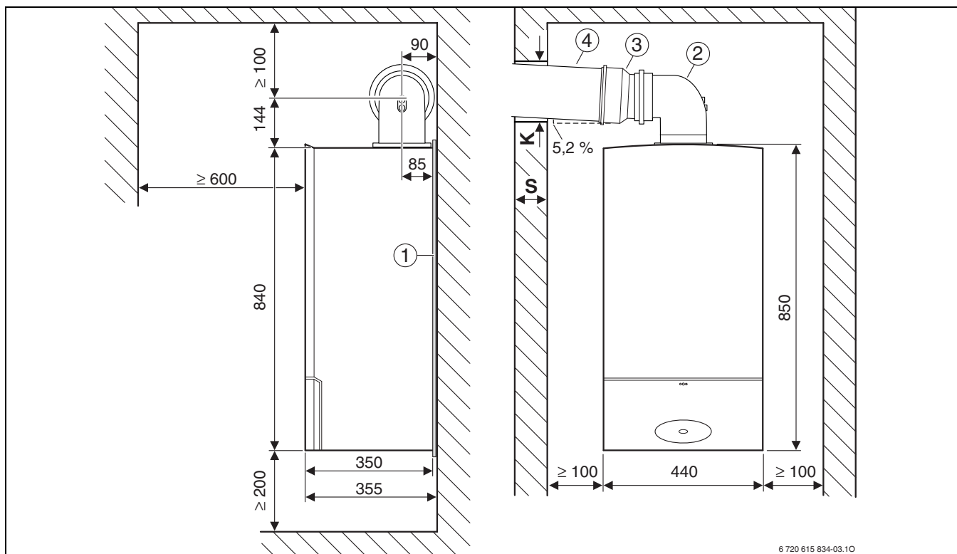
Рис 6 Отвод дымовых газов Ø 100/150 мм
