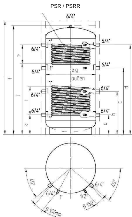
Емкости PSR / PSRR со спиральным ТО PSR 500 – 5000 л PSRR 500 – 3000 л
